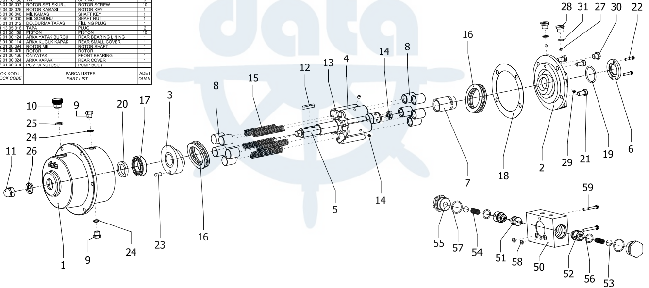
DP 63 - DP 63K HİDROLİK EL POMPASI (HYDRAULIC HELM PUMP)
