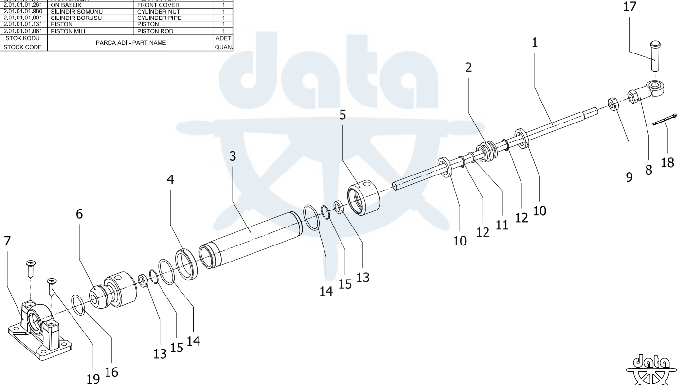
DS 50 HİDROLİK SİLİNDİR (HYDRAULIC CYLINDER)
